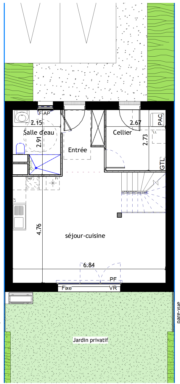
Rez de Chaussée
